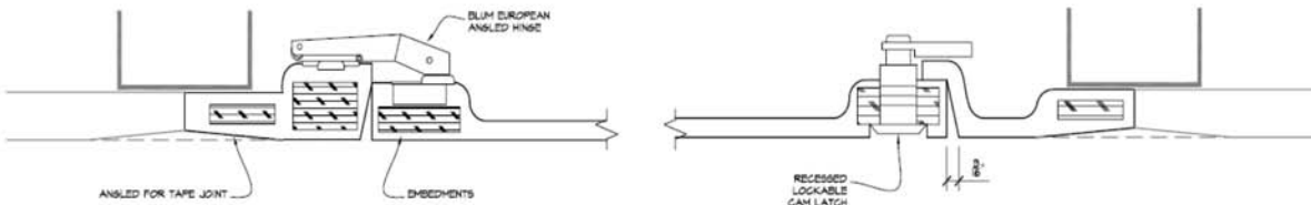
SECTION VIEW Scale: 6"=1'
